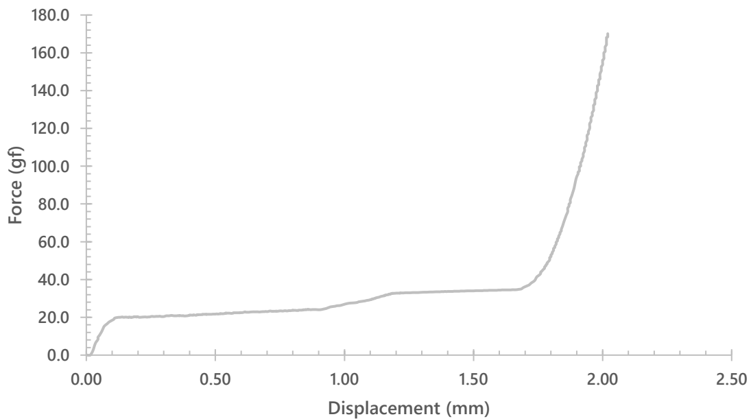
Kailh Black Kite Mini (Upstroke)
